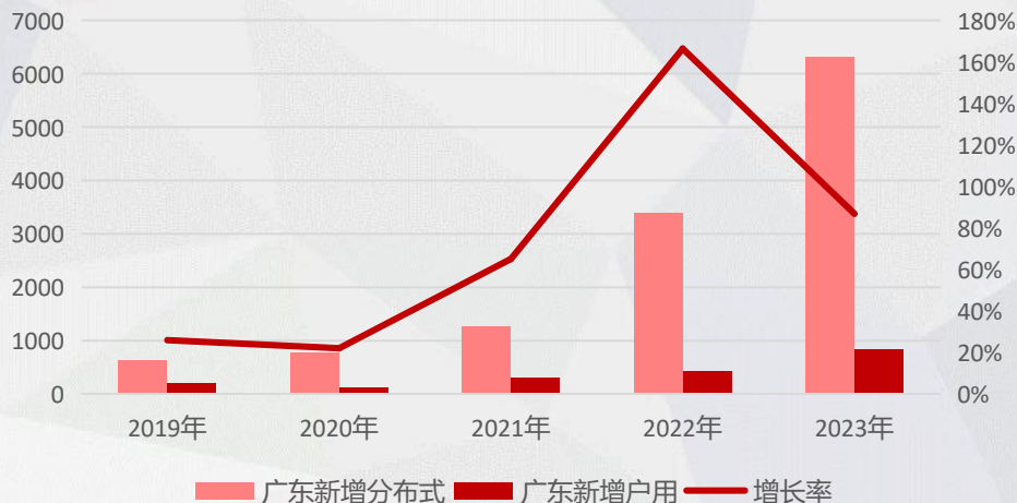
广东省分布式光伏装机与增长 (MW)
